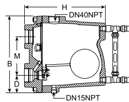
图LD-46. JD和KD系列
