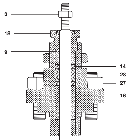
带石墨密封阀帽
