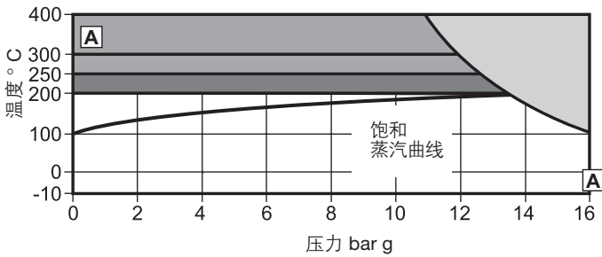
法兰 EN 1092 PN16
