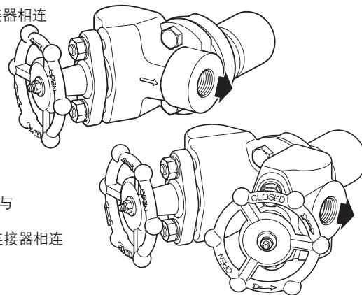
USM21 与 PC3 管道连接器相连
