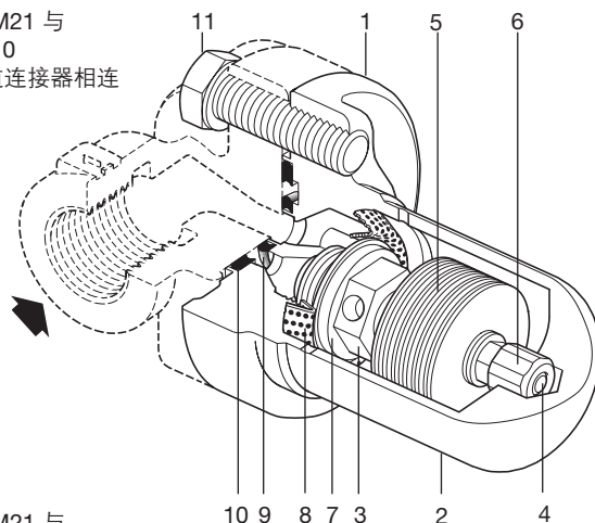
USM21 与 PC3 管道连接器相连
