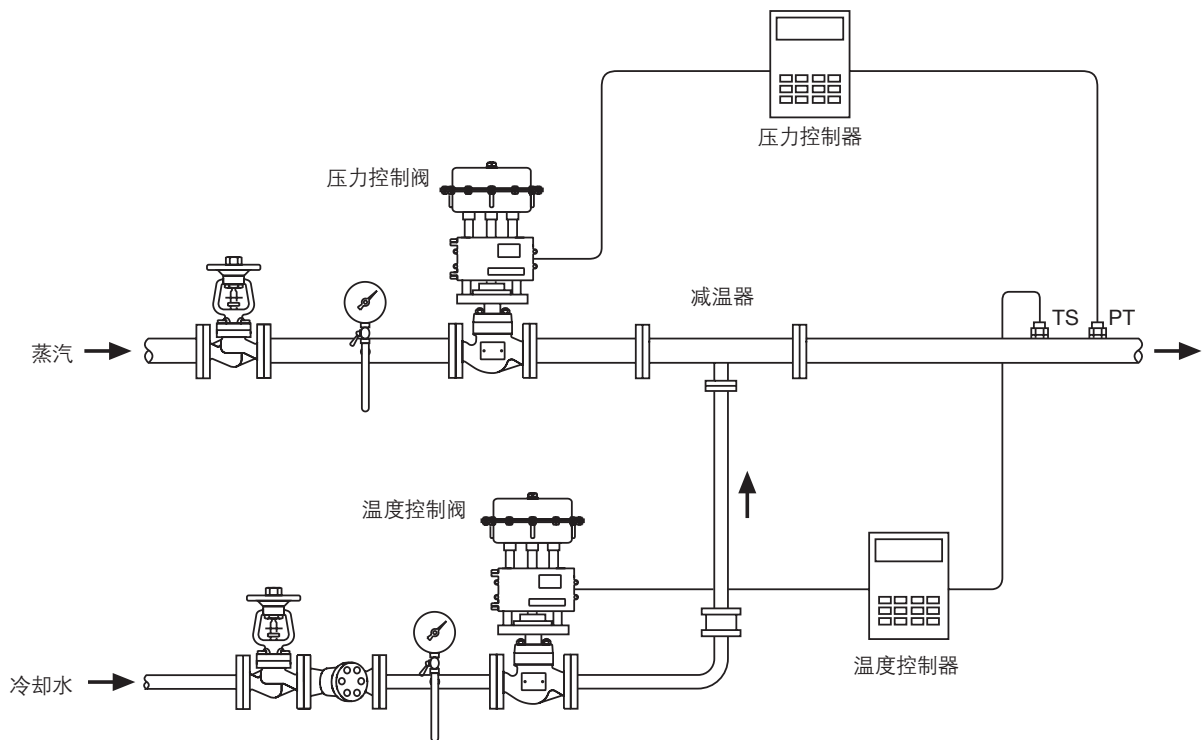
喷雾型和文丘利型减温器的减温和减压系统典型布置
