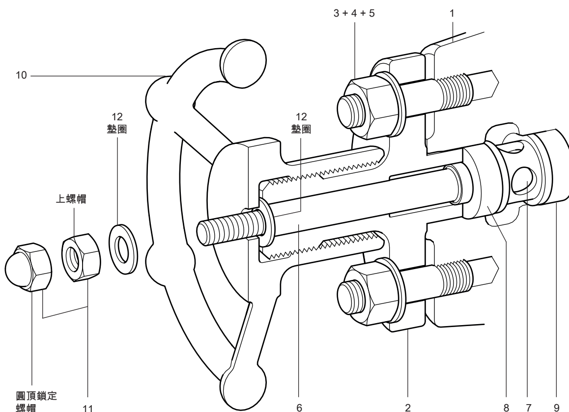
拔出工具
