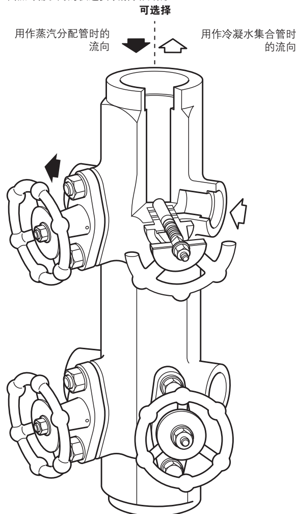
图示为MSC04 承插焊连接
