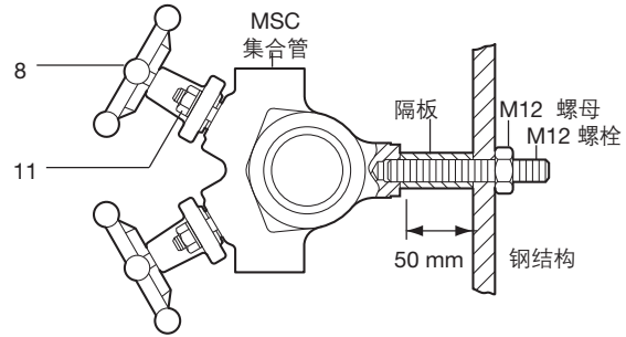
安装俯视图示意图
