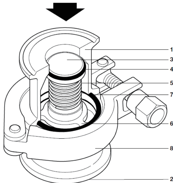
图示为1" 阀门
