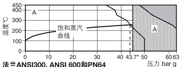
法兰ANSI300, ANSI 600和PN64
