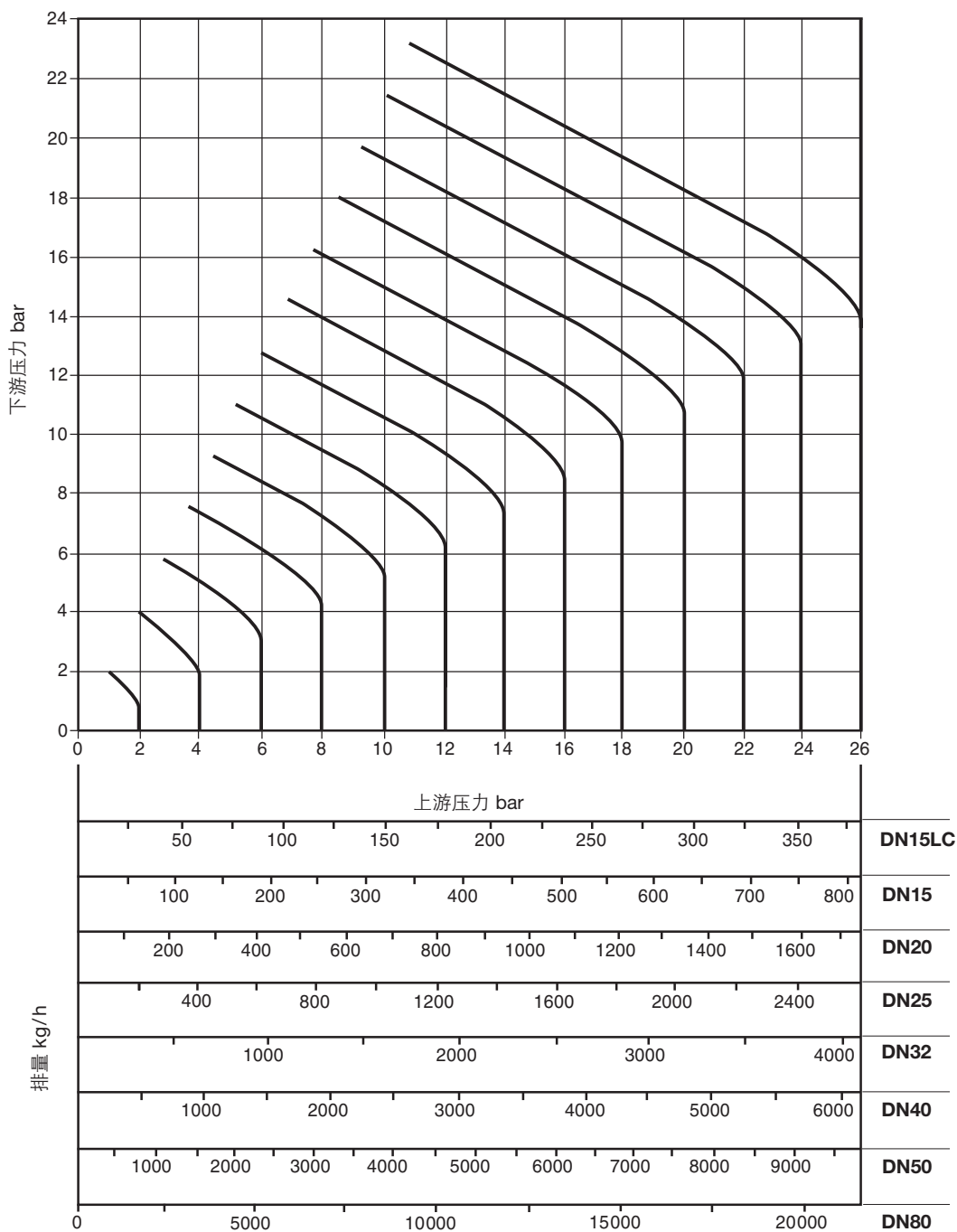
蒸汽排量图
