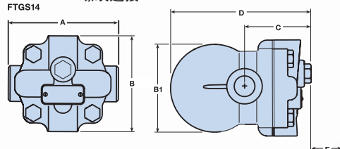
螺纹连接
