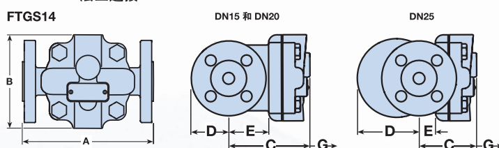
法兰连接
