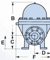
FT450 (DN80/DN100)
