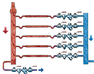
从压烫机中排放冷凝水
