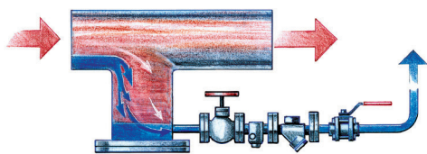
从蒸汽主管排放冷凝水
